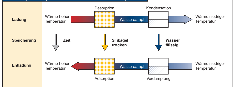
Abb 3 Speicherzyklus eines thermochemischen Speichers
